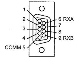
RS-485 DB9-F
