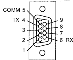
RS-232 DB9-M
