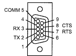
RS-232 DB9-M
