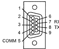
RS-232 DB9-F
